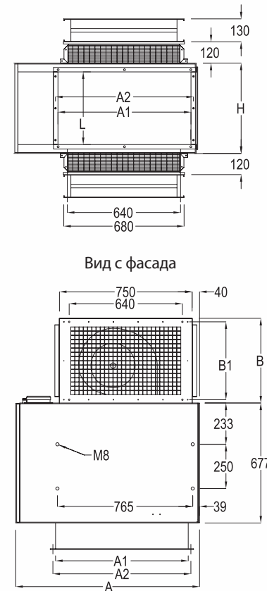
Вид снизу Без клапана воздушного
