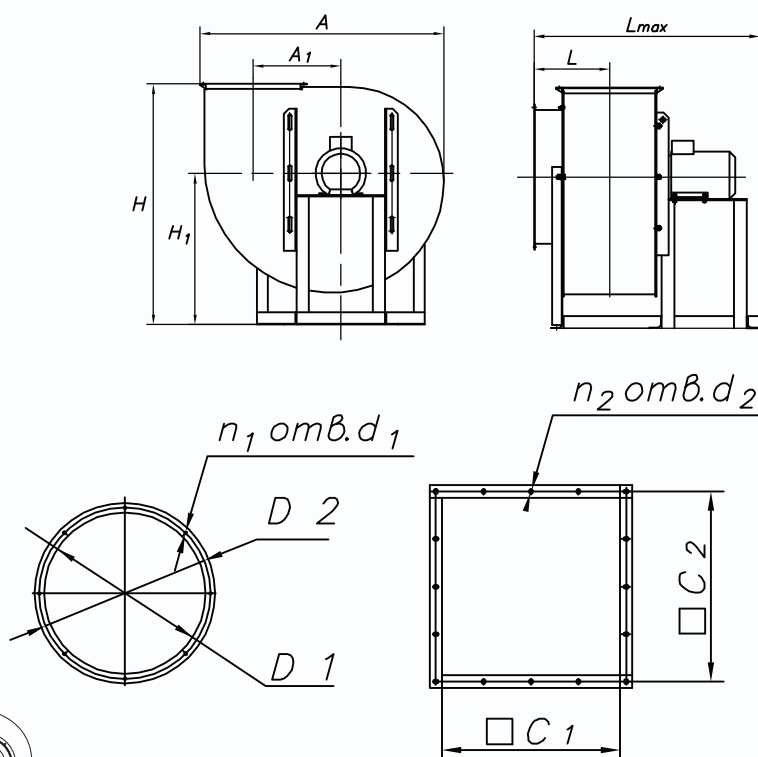
Общий вид и размеры вентилятора
