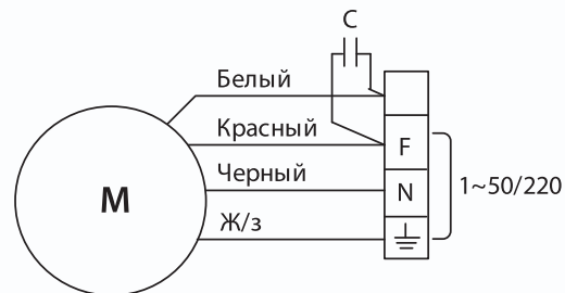
Электрическая схема
