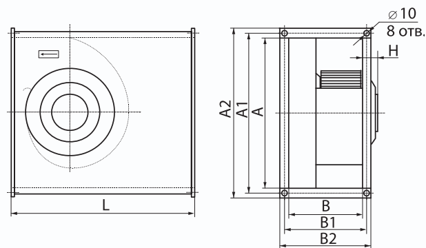
Общий вид и размеры вентилятора
