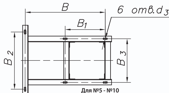
Схема расположений отверстий под фундаментные болты
