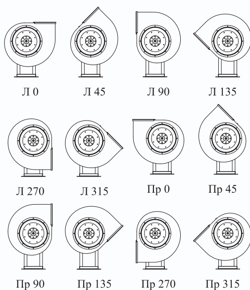
Вид со стороны всасывания
