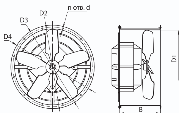
Общий вид и размеры вентилятора
