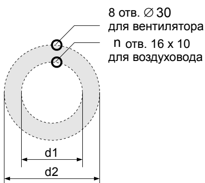
Крепление вентилятора ВКР 3,15 .. 6,3 Крепление вентилятора ВКР 8 .. 10
