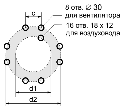
Крепление вентилятора ВКР 12,5
