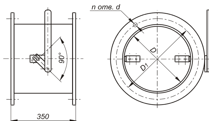
Габаритные и присоединительные размеры заслонки АЗД - 196, АЗД - 197
