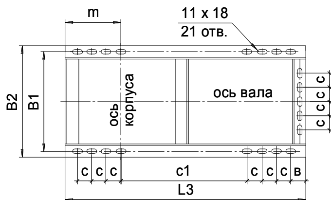
Расположение отверстий крепления вентиляторов 2 .. 6,3
