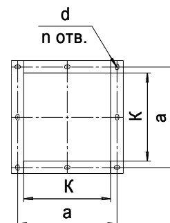
Расположение отверстий крепления вентиляторов 10 .. 12,5
