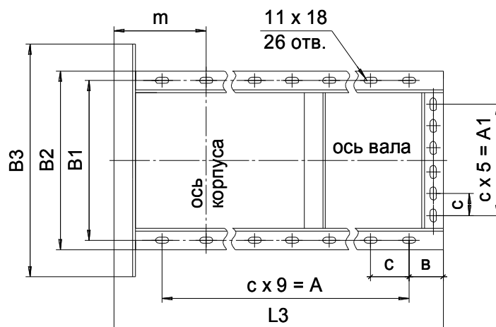
Расположение отверстий крепления вентиляторов 10 .. 12,5
