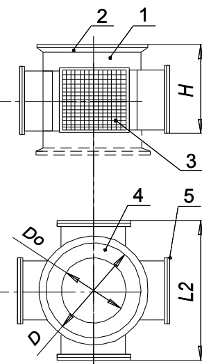
Четырехструйный воздухораспределитель
