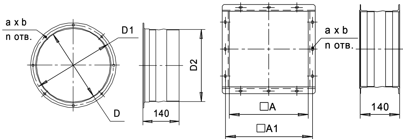
Габаритные и присоединительные размеры гибких вставок
