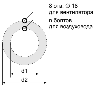
Крепление вентилятора ВКР 3,15 .. 6,3 Крепление вентилятора ВКР 8 .. 10
