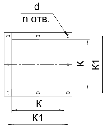
Расположение отверстий крепления вентиляторов 10 .. 12,5
